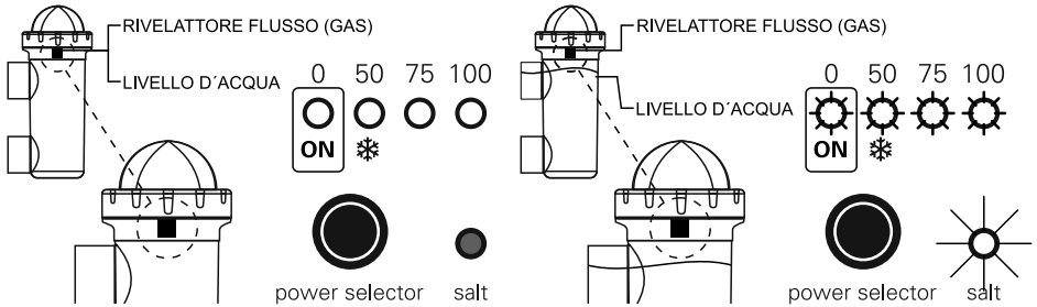
1. Rivelatore di gas sommerso. Sistema operativo.
